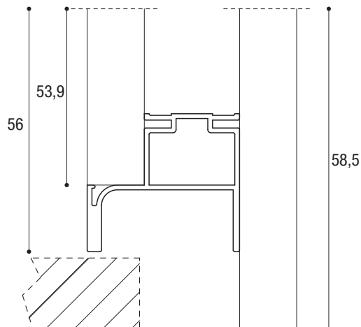
GOLA "J" ALLUMINIO
