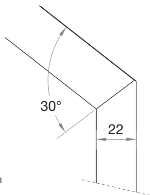
Sezione anta Door section Section porte Sección de la puerta
