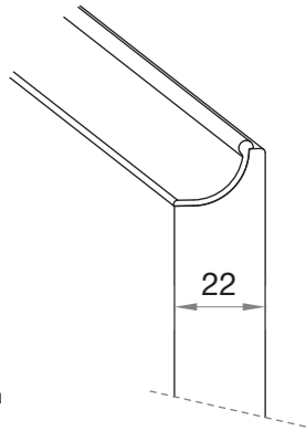
Sezione anta Door section Section porte Sección de la puerta
